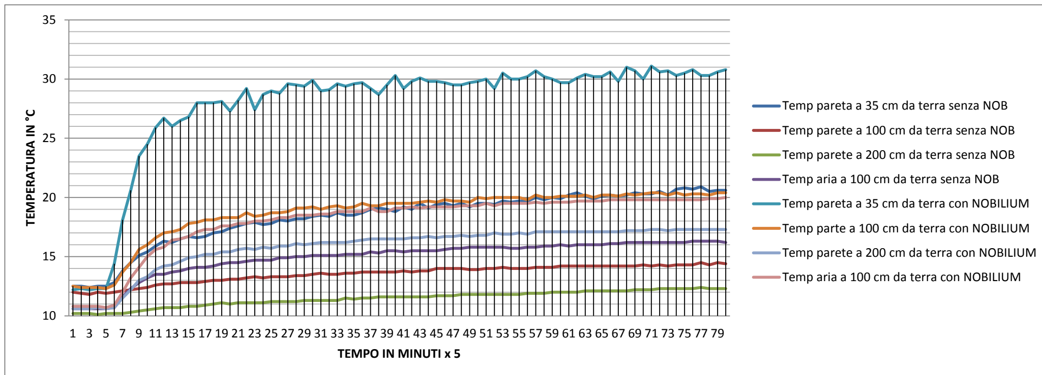
GRAFICO DI ANALISI TEMPERATURE PARETE CON E SENZA NOBILIUM®THERMALPANEL DA 9MM
